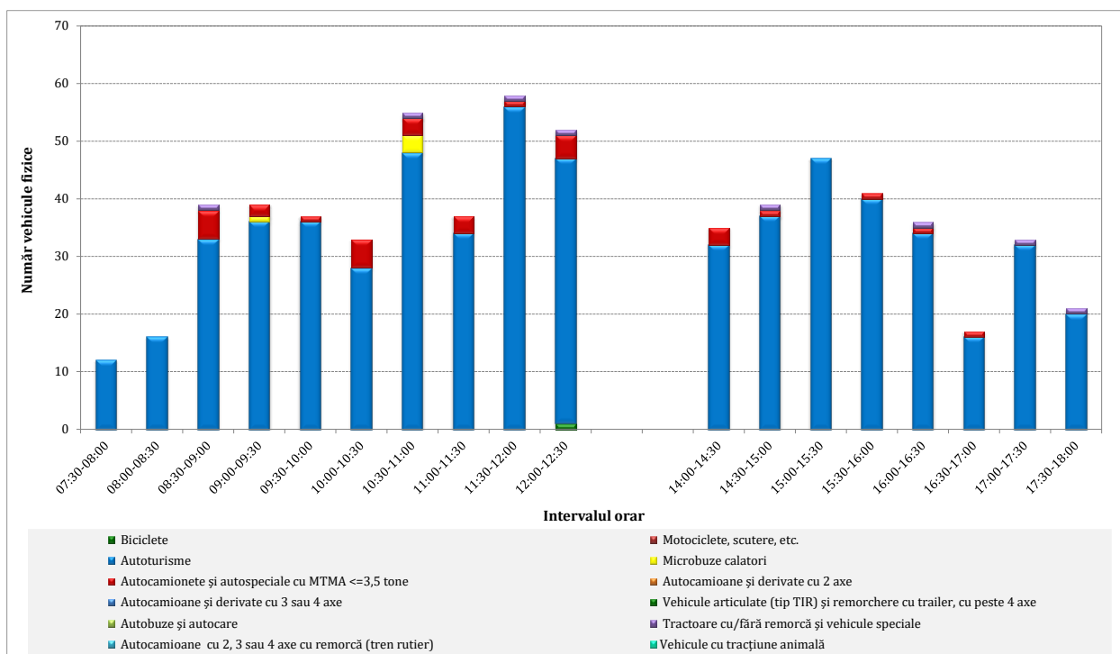
Figura 3.7. Distribuția volumelor de trafic. Postul 1, braț 3 -Str. Tudor Vladimirescu Est.
