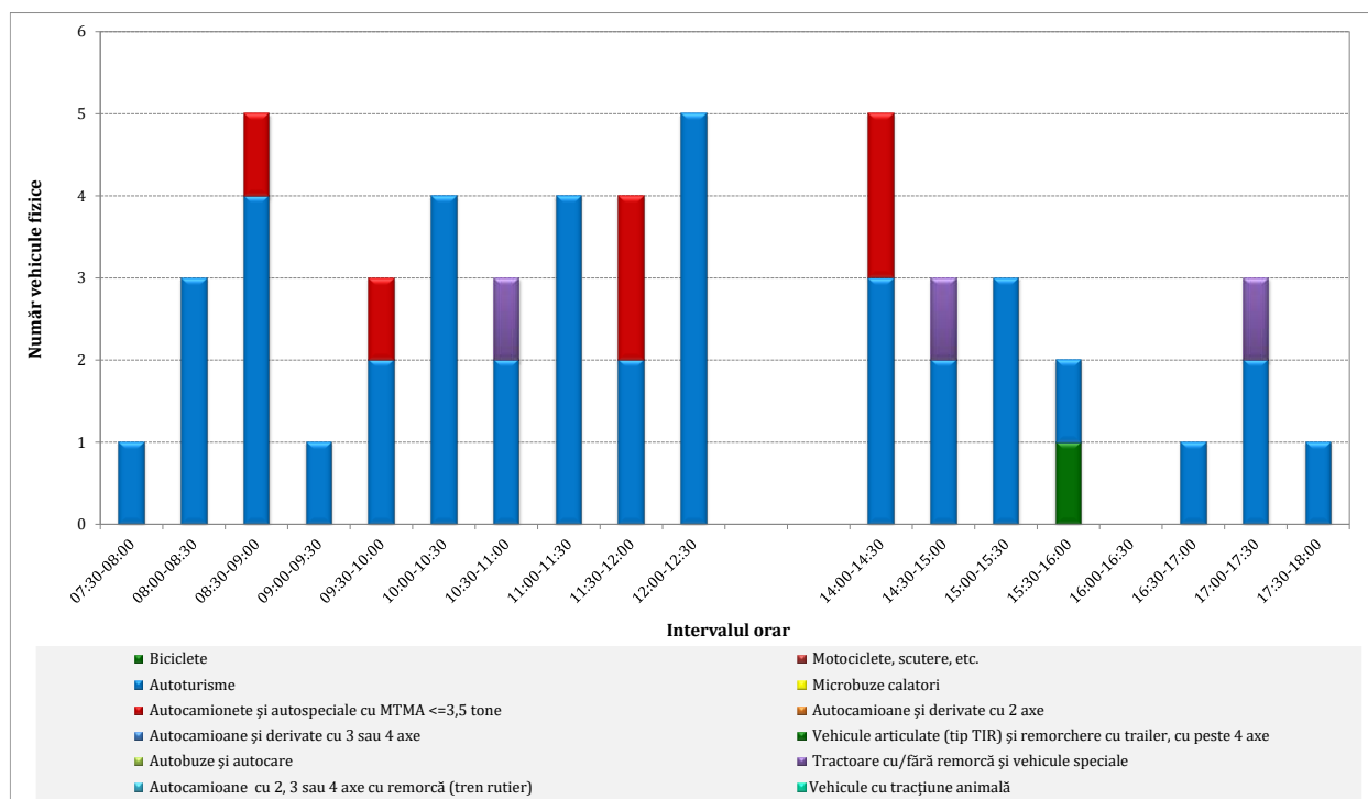
Figura 3.8. Distribuția volumelor de trafic. Postul 1, braț 4 – Str. Sfatului.
