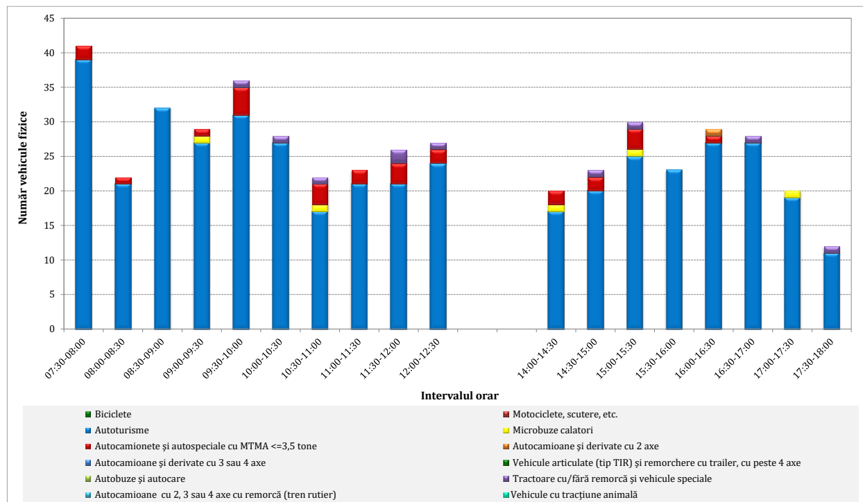
Figura 3.5. Distribuția volumelor de trafic. Postul 1, braț 1 -Str. Tudor Vladimirescu Nord.
