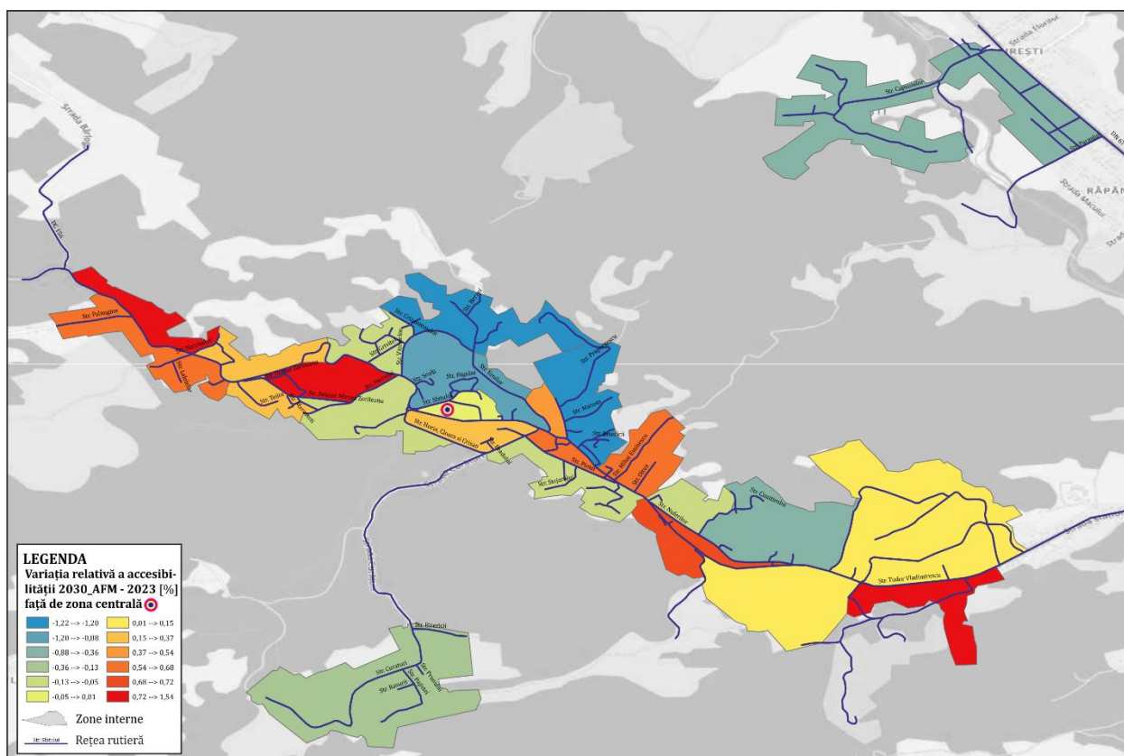
Figura 4.10. Variația relativă a accesibilității, scenariul "A face minim" 2030 vs. Anul de bază 2023, față de zona centrală.
