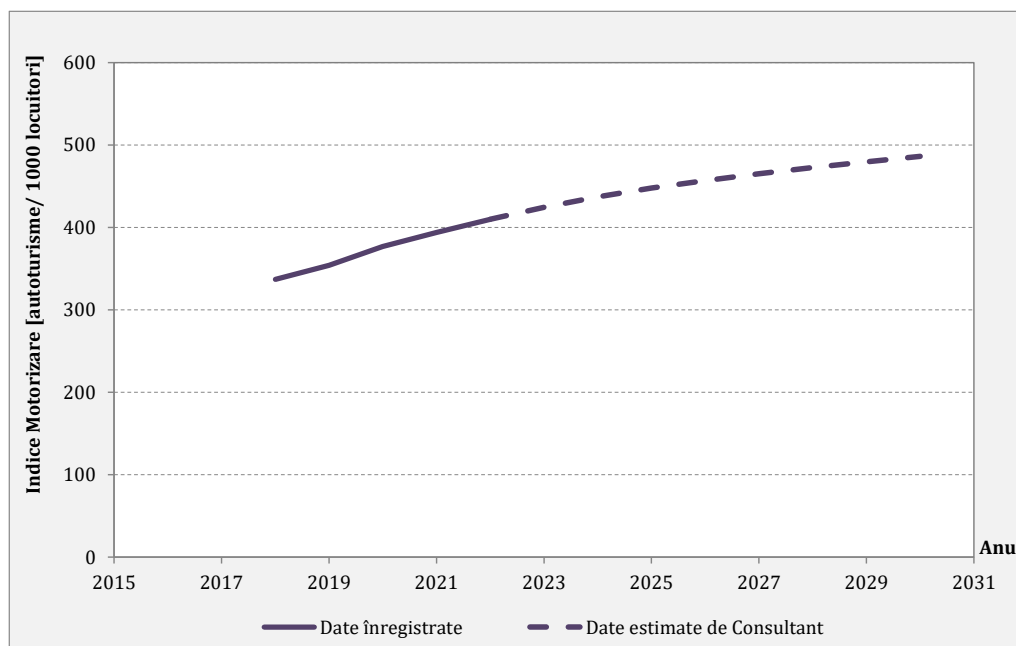
Figura 3.32. Prognoza indicelui de motorizare – Orașul Băile Govora.
