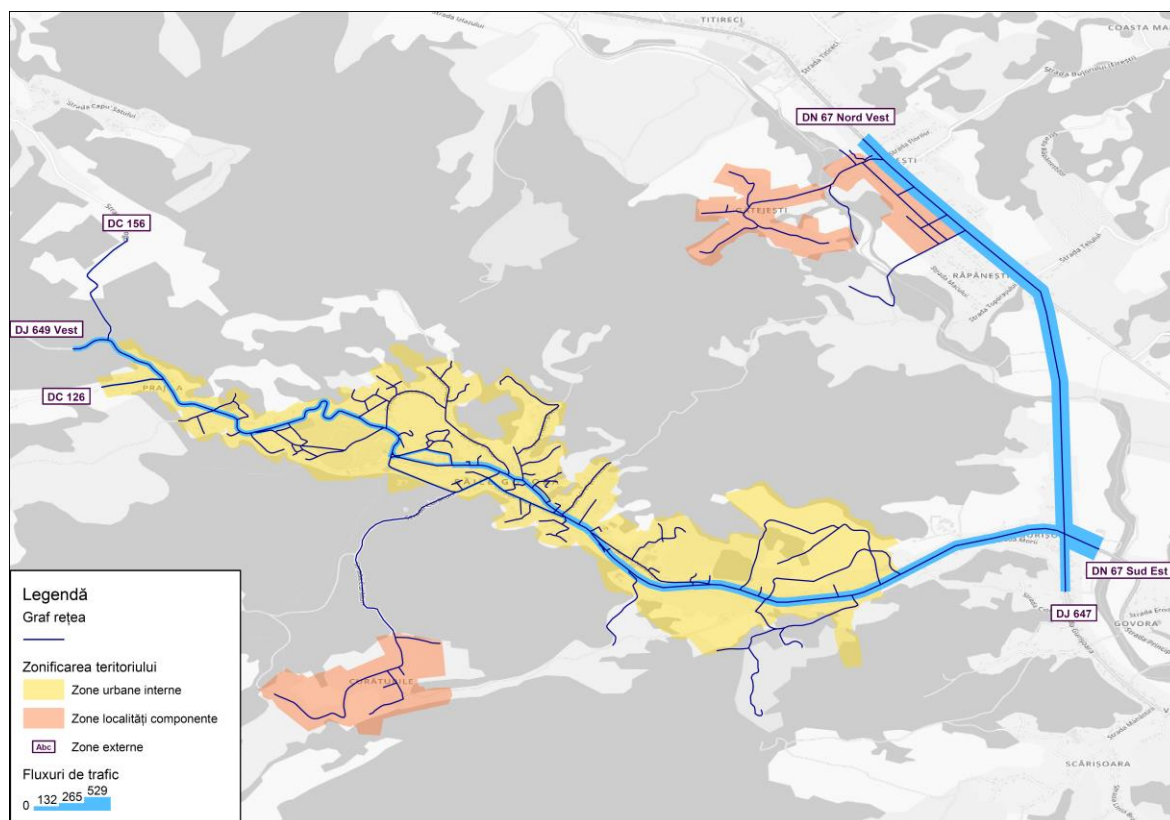
Figura 3.24. Fluxuri de trafic, vehicule etalon, ora de varf de trafic, 2023.
