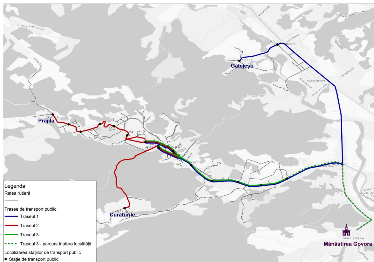
Figura 2.1. Trasee transport public local în Orașul Băile Govora - Propunere.
