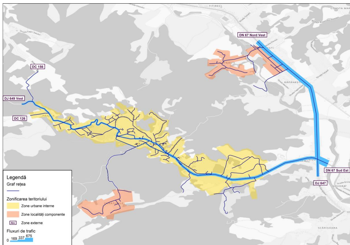
Figura 3.35. Fluxuri de trafic, vehicule etalon, Scenariul AFM_ ora de vârf de trafic, 2030.
