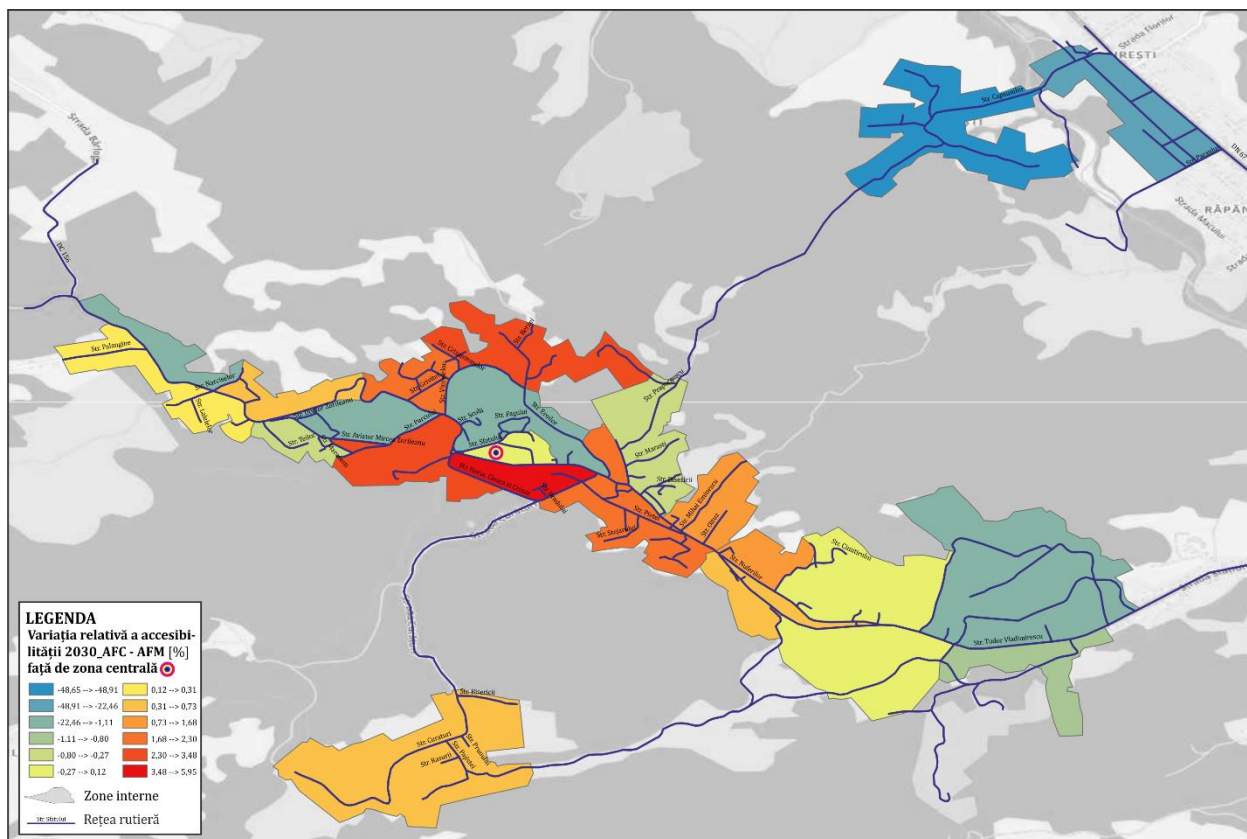
Figura 7.2. Variația relativă a accesibilității față de Zona Centrală, scenariul AFC 2030 vs. scenariul AFM 2030.
