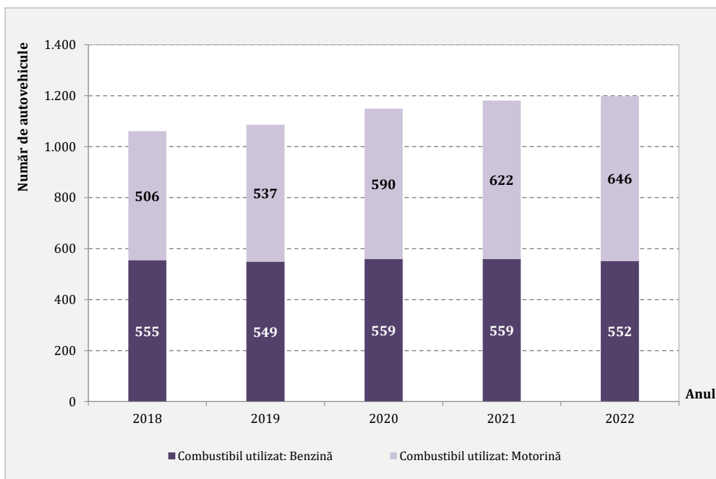
Figura 4.3. Situația parcului inventar de autovehicule în funcție de combustibilul utilizat – Orașul Băile Govora. Sursa datelor: Direcția Regim Permise Conducere și Înmatriculare a Vehiculelor, București.
