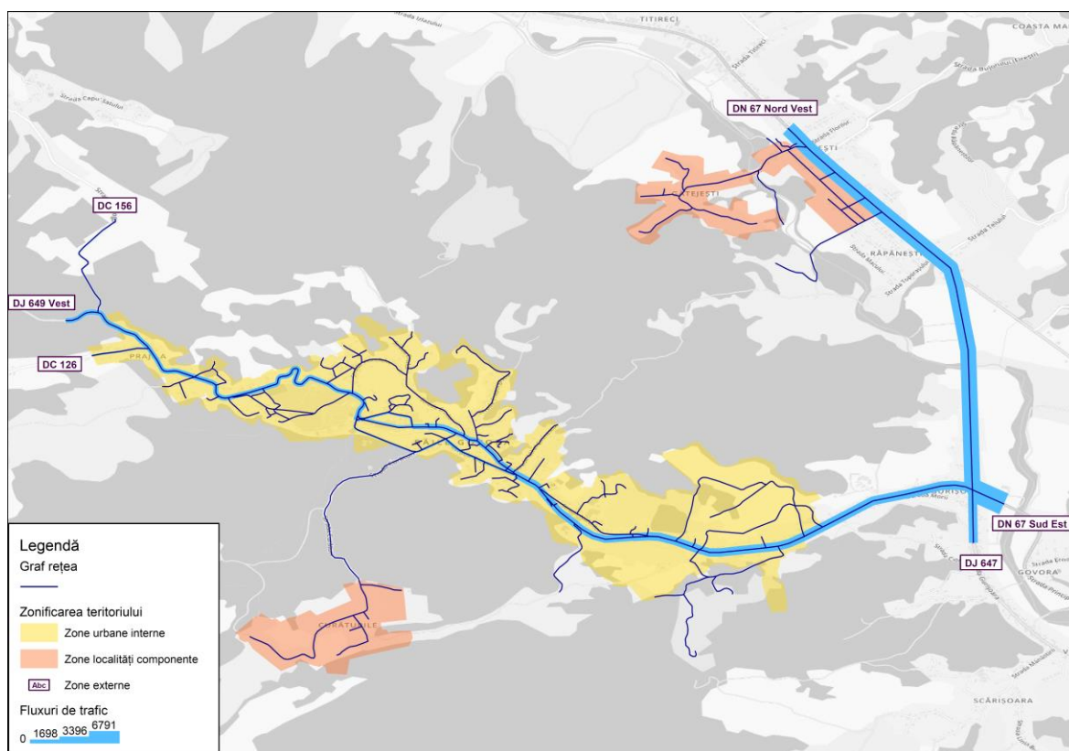
Figura 3.36. Fluxuri de trafic, autovehicule etalon, Scenariul ANFN_MZA, 2030.
