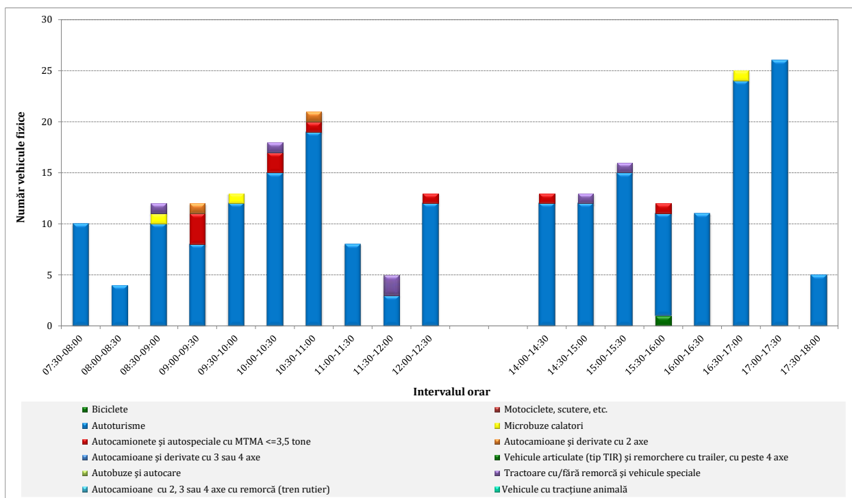
Figura 3.6. Distribuția volumelor de trafic. Postul 1, braț 2 -Str. Horea, Cloșca și Crișan.
