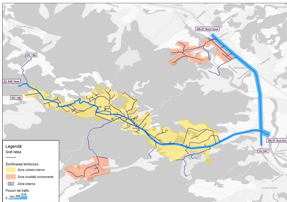
Figura 3.37. Fluxuri de trafic, vehicule etalon, Scenariul ANFN_ ora de vârf de trafic, 2030.
